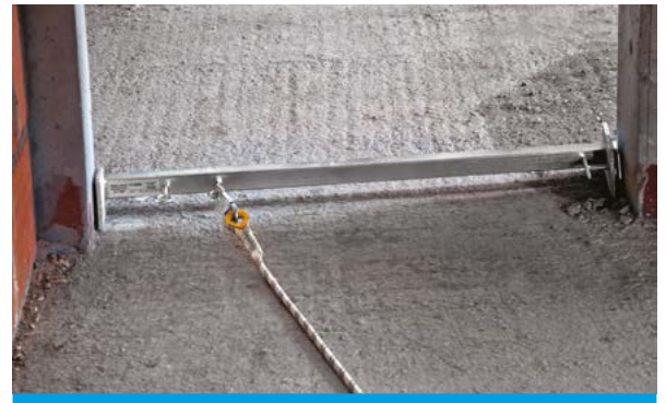
Kotwienie do belki poprzecznej mocowanej w otworach ściennych.
