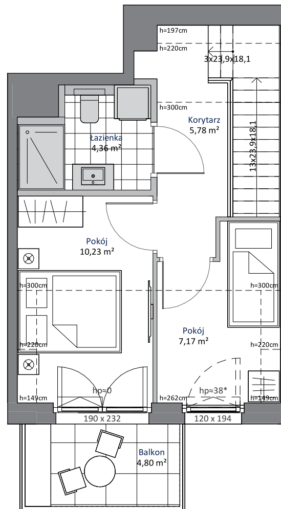
Poziom 2
